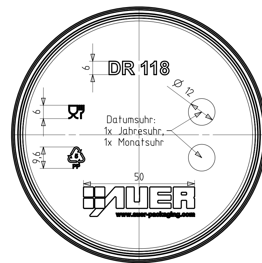
Ansicht Deckel von unten
